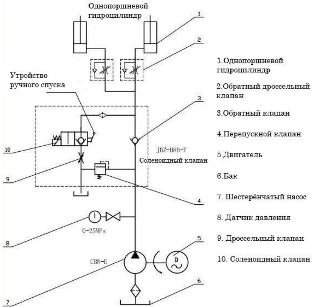
Рисунок 3. Схема гидравлическая
