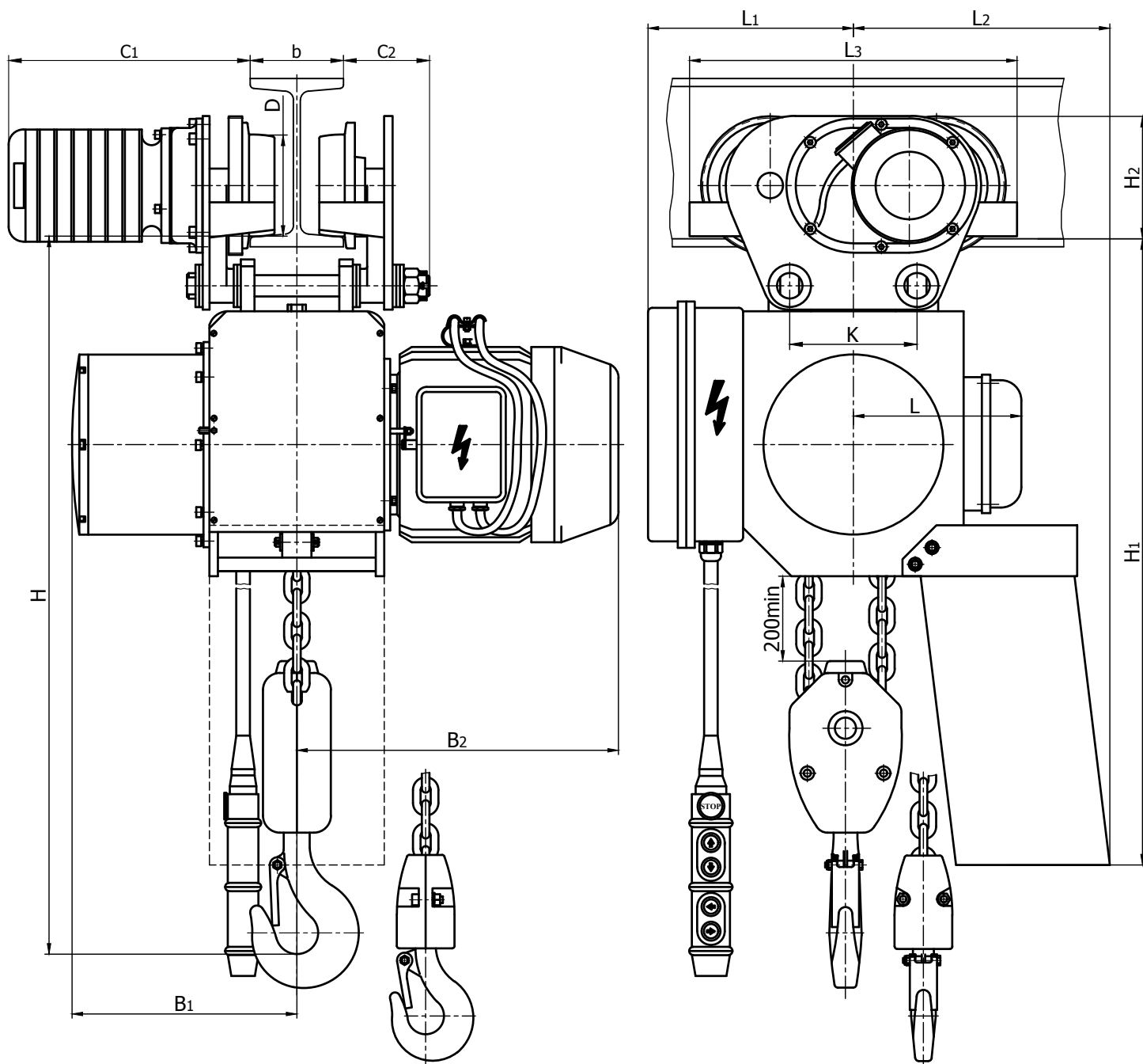
ЦЕПНАЯ ЭЛЕКТРОТАЛЬ ТИПА ВУ...(М) НА ЭЛЕКТРИЧЕСКОЙ ТЕЛЕЖКЕ
